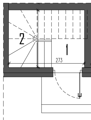
RZUT PARTERU
