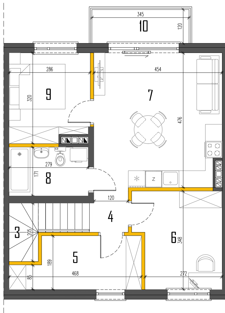
RZUT PIĘTRA
