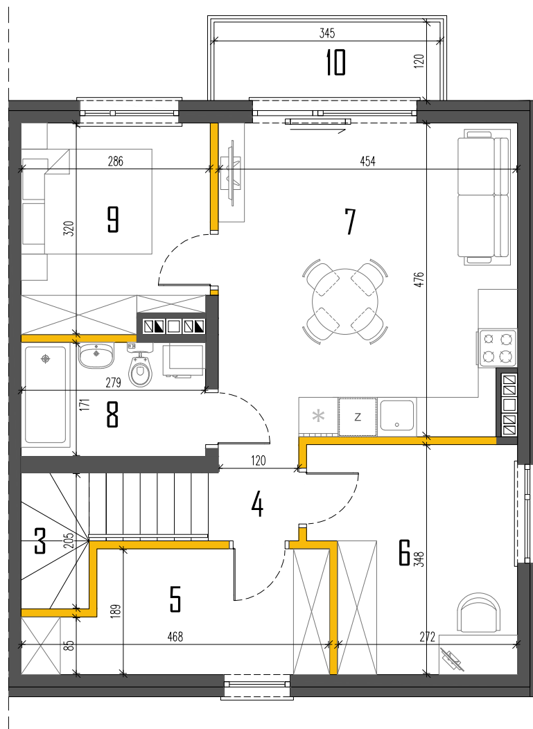
RZUT PIĘTRA
