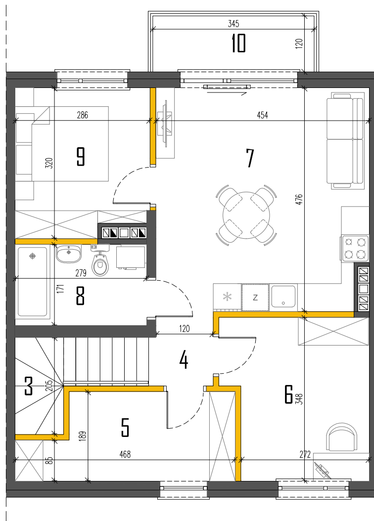
RZUT PIĘTRA
