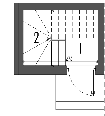
RZUT PARTERU
