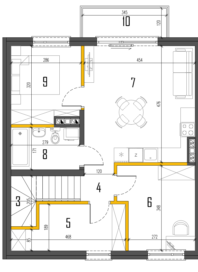
RZUT PIĘTRA
